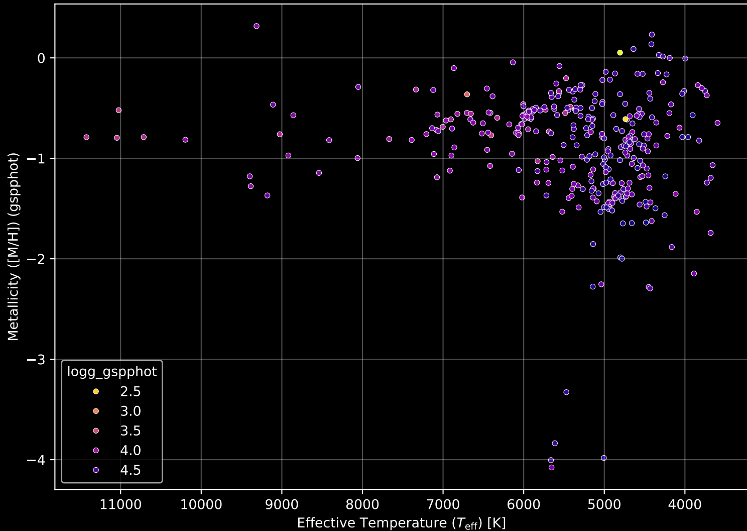
Gaia Cluster: [ASCC_88] Stellar Population Parameters (n= 324)
