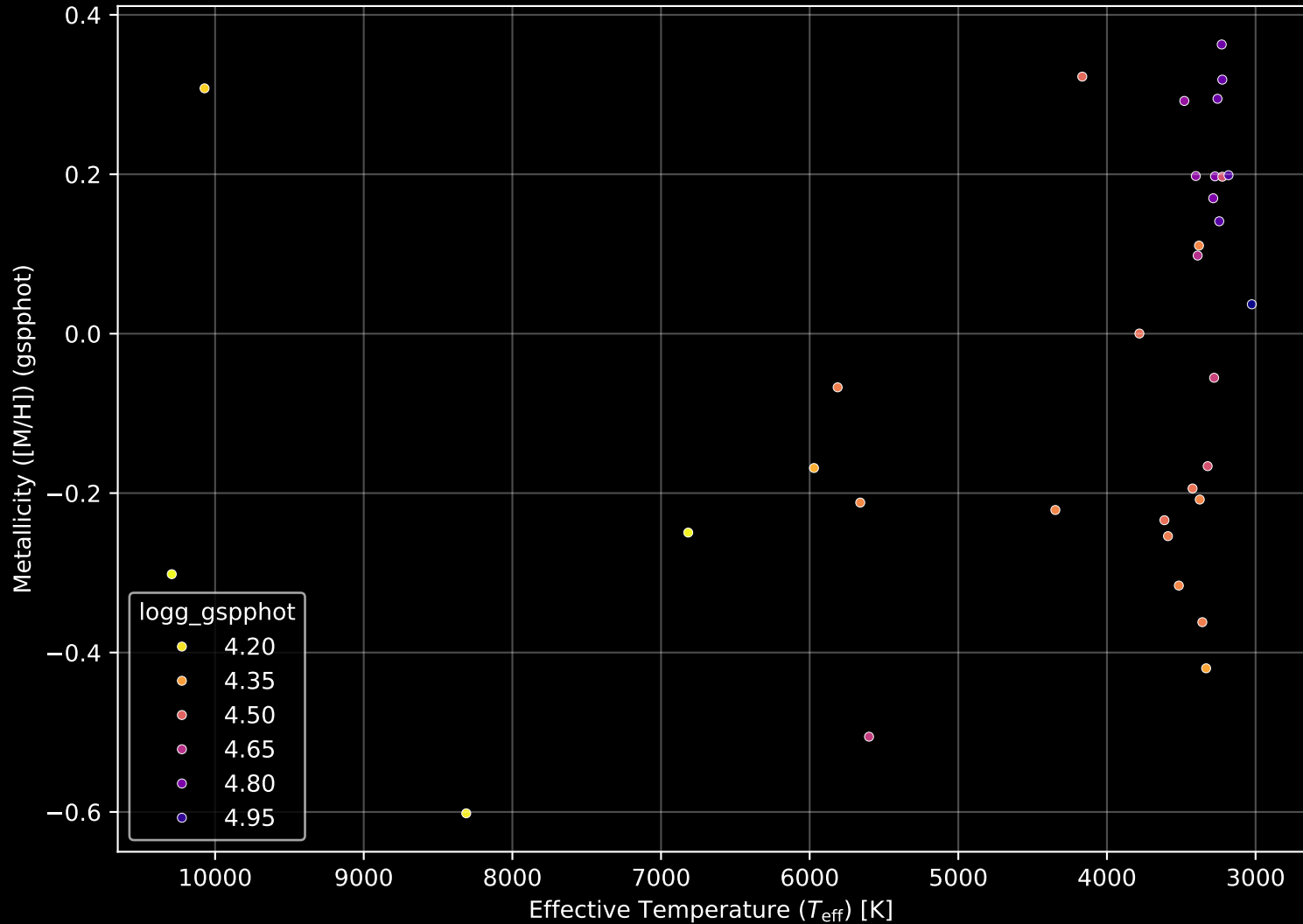
Gaia Cluster: [Alessi 13] Stellar Population Parameters (n= 33)
