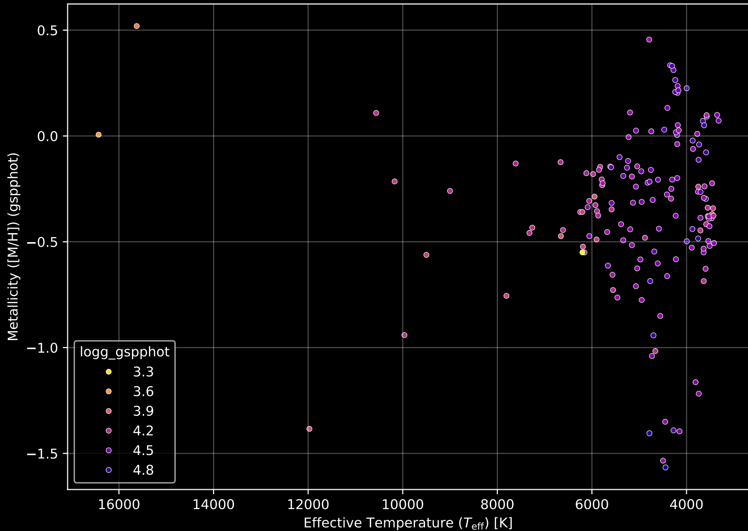
Gaia Cluster: [Alessi_19] Stellar Population Parameters (n= 156)
