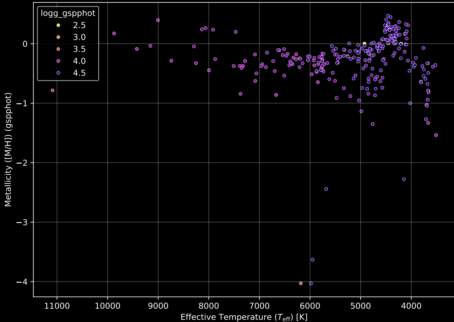
Gaia Cluster: [Alessi_2] Stellar Population Parameters (n= 247)
