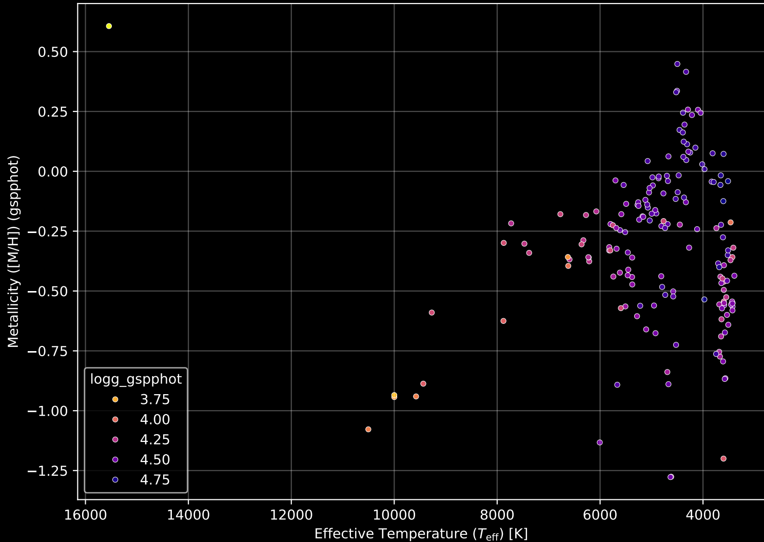
Gaia Cluster: [Alessi_24] Stellar Population Parameters (n= 172)
