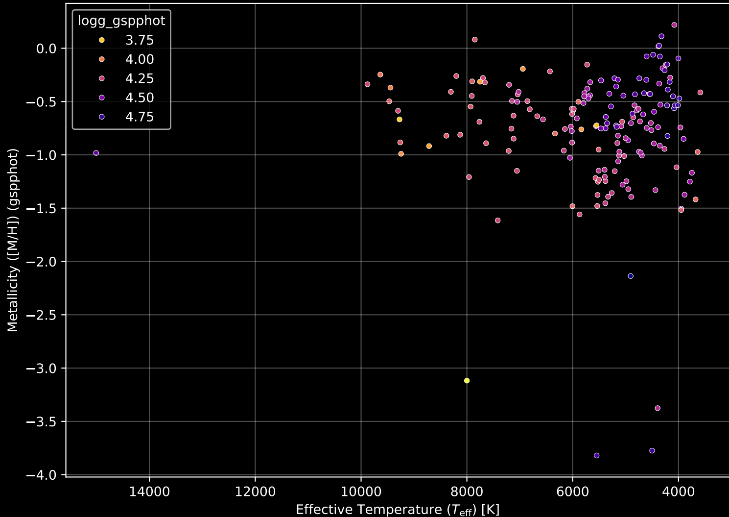
Gaia Cluster: [Alessi_31] Stellar Population Parameters (n= 176)
