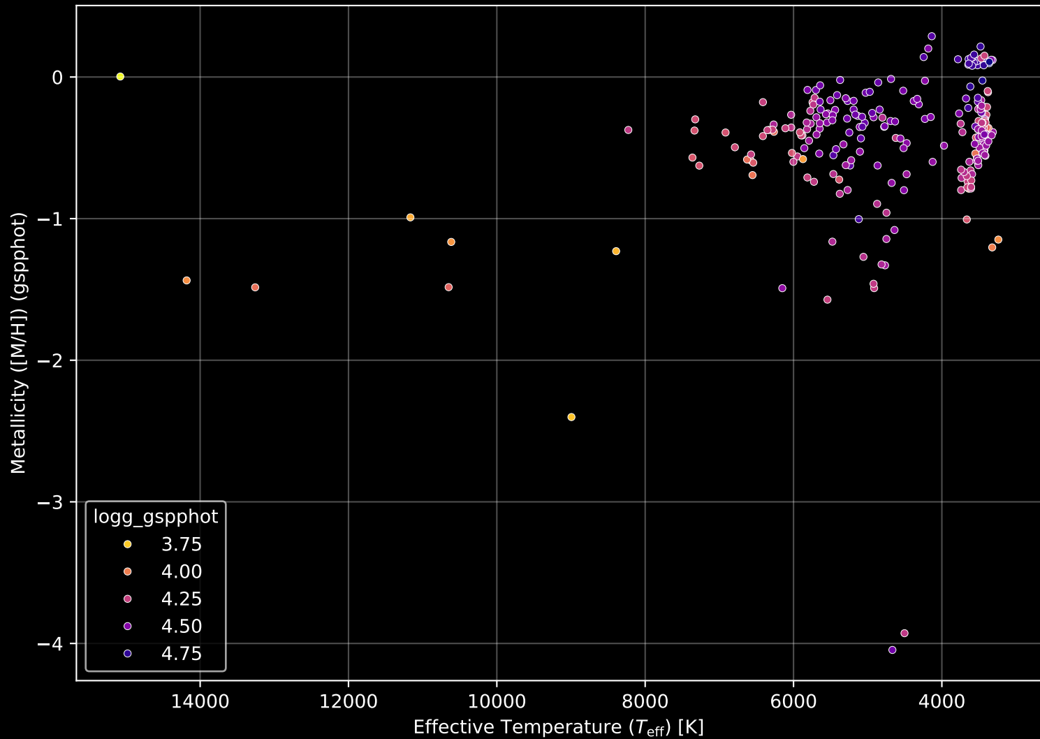
Gaia Cluster: [Alessi_5] Stellar Population Parameters (n= 250)
