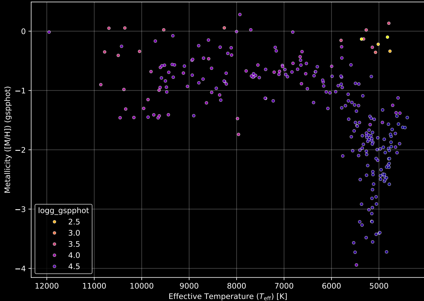
Gaia Cluster: [Alessi_60] Stellar Population Parameters (n= 255)
