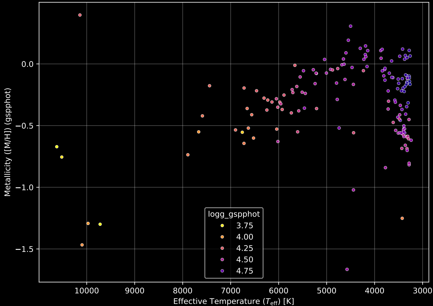
Gaia Cluster: [Alessi_9] Stellar Population Parameters (n= 157)
