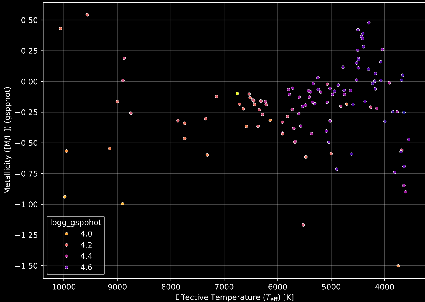
Gaia Cluster: [Alessi_Teutsch_11] Stellar Population Parameters (n= 118)
