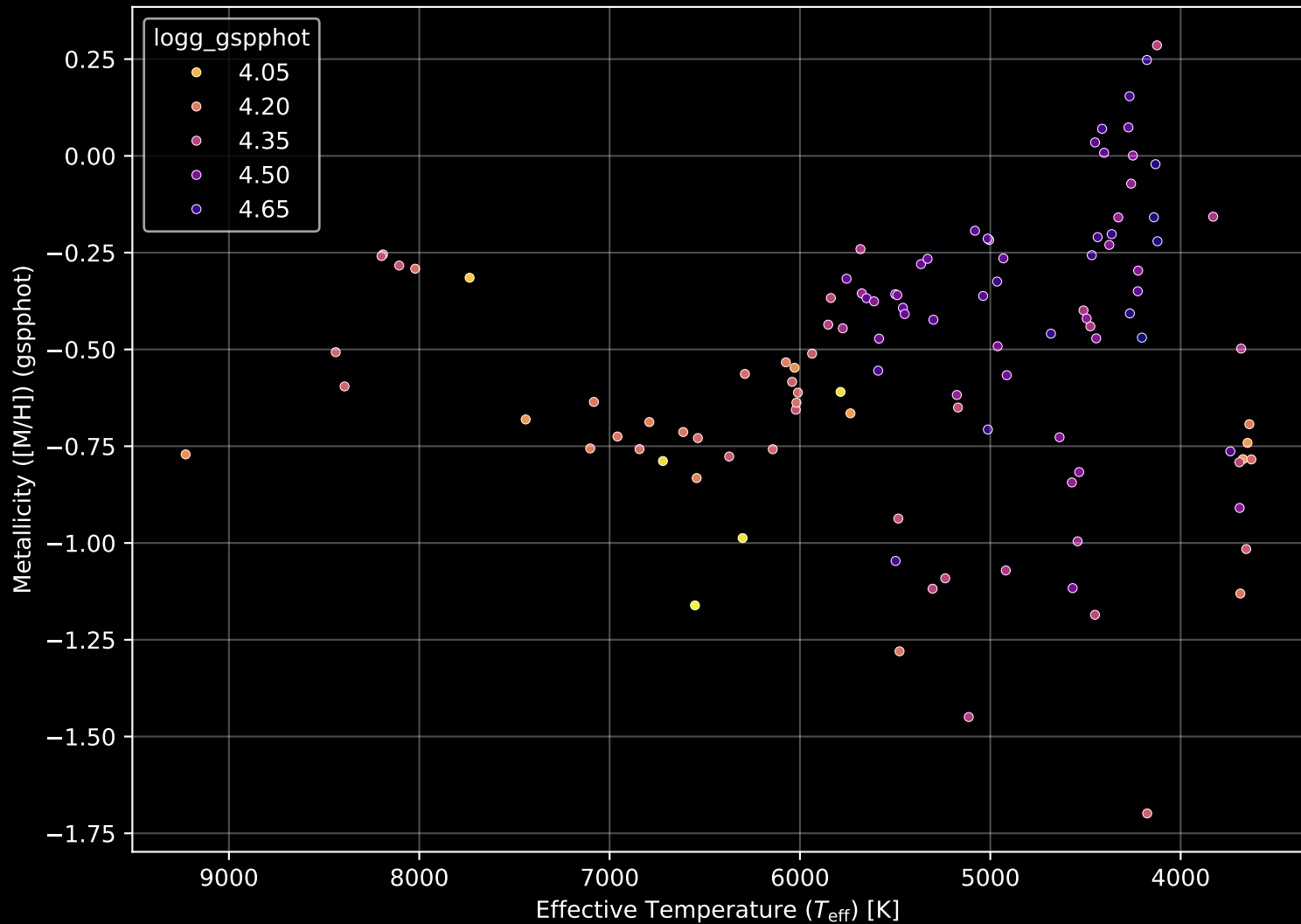
Gaia Cluster: [Alessi_Teutsch_3] Stellar Population Parameters (n= 111)
