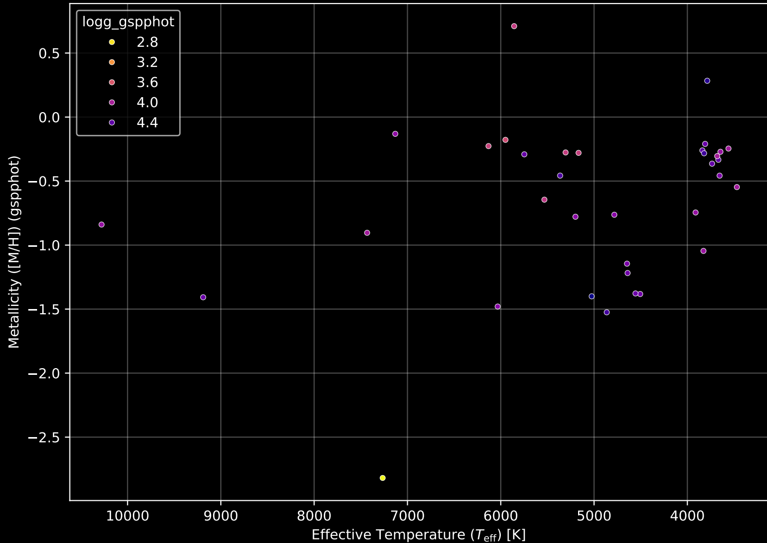
Gaia Cluster: [Antalova_2] Stellar Population Parameters (n= 35)
