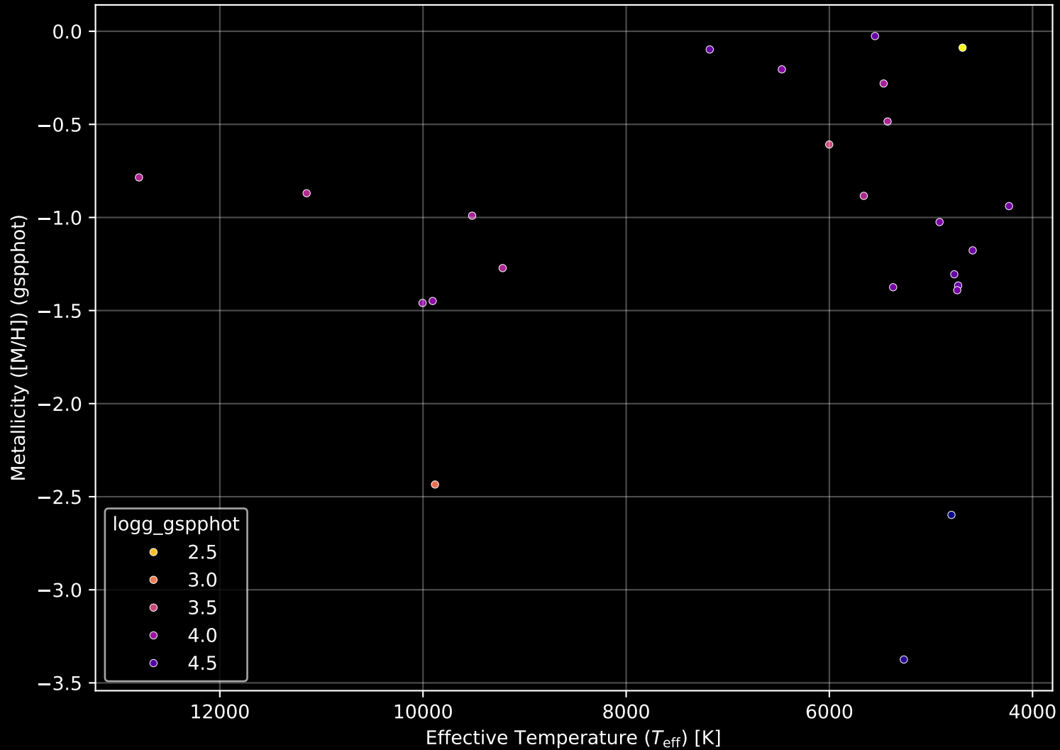
Gaia Cluster: [BDSB93] Stellar Population Parameters (n= 24)
