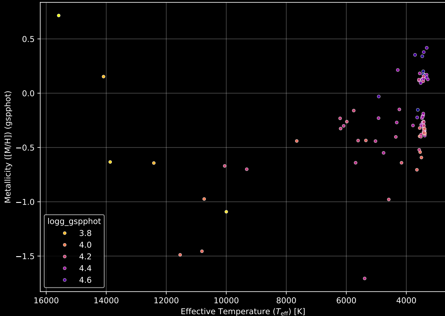
Gaia Cluster: [BH_23] Stellar Population Parameters (n= 94)
