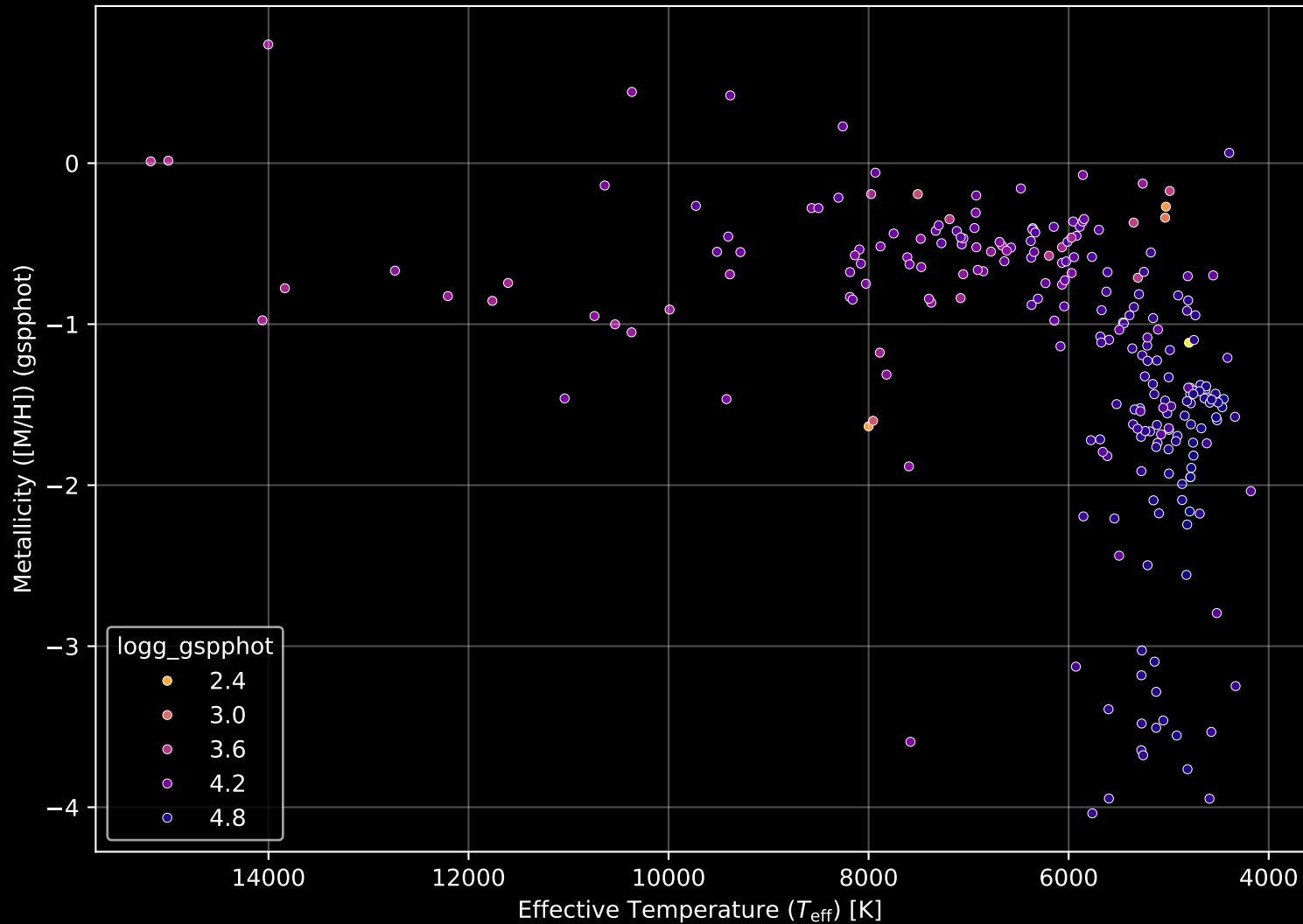
Gaia Cluster: [Basel_17] Stellar Population Parameters (n= 239)
