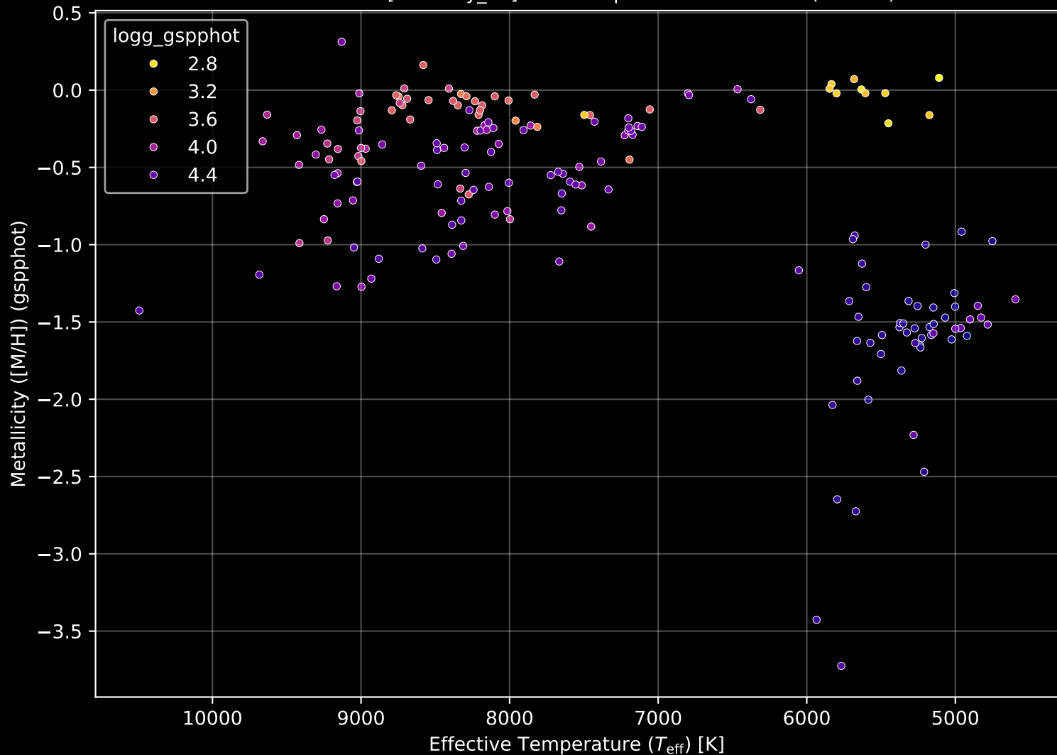
Gaia Cluster: [Berkeley_10] Stellar Population Parameters (n= 186)
