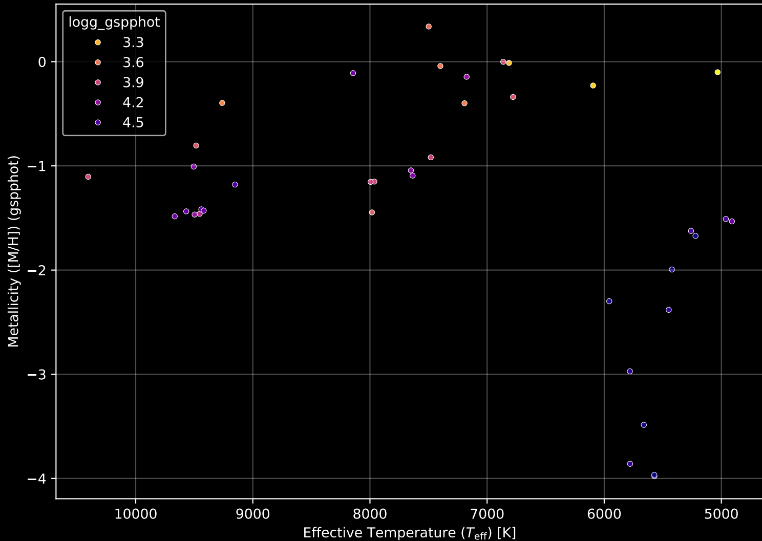
Gaia Cluster: [Berkeley_100] Stellar Population Parameters (n= 39)
