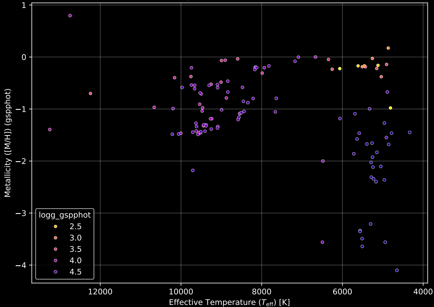
Gaia Cluster: [Berkeley_104] Stellar Population Parameters (n= 121)
