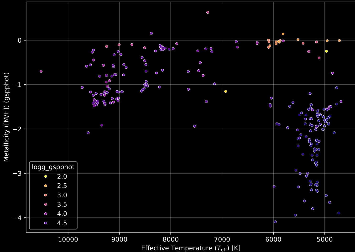
Gaia Cluster: [Berkeley_13] Stellar Population Parameters (n= 237)
