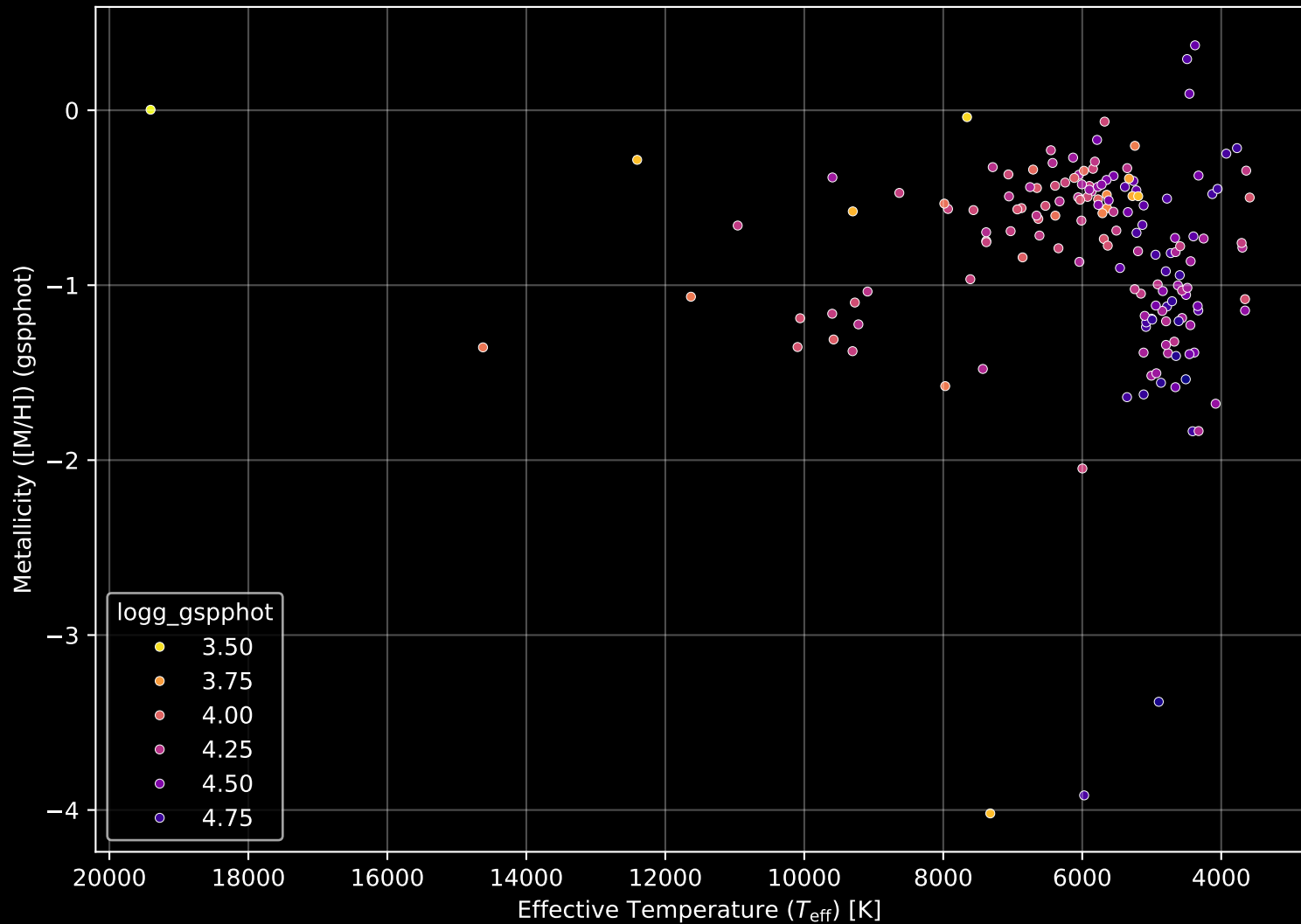
Gaia Cluster: [Berkeley_14A] Stellar Population Parameters (n= 162)
