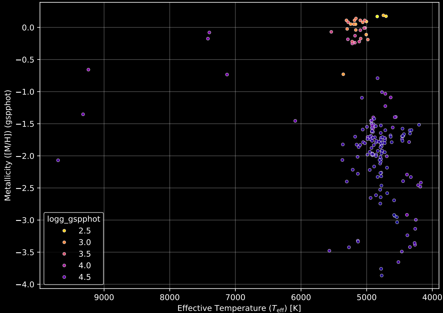
Gaia Cluster: [Berkeley_17] Stellar Population Parameters (n= 181)
