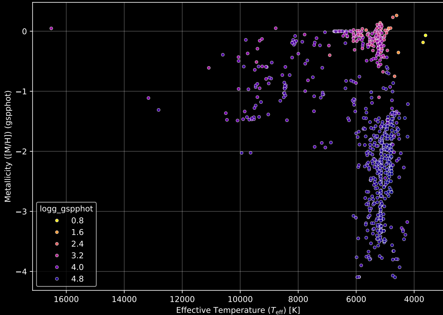
Gaia Cluster: [Berkeley_18] Stellar Population Parameters (n= 712)
