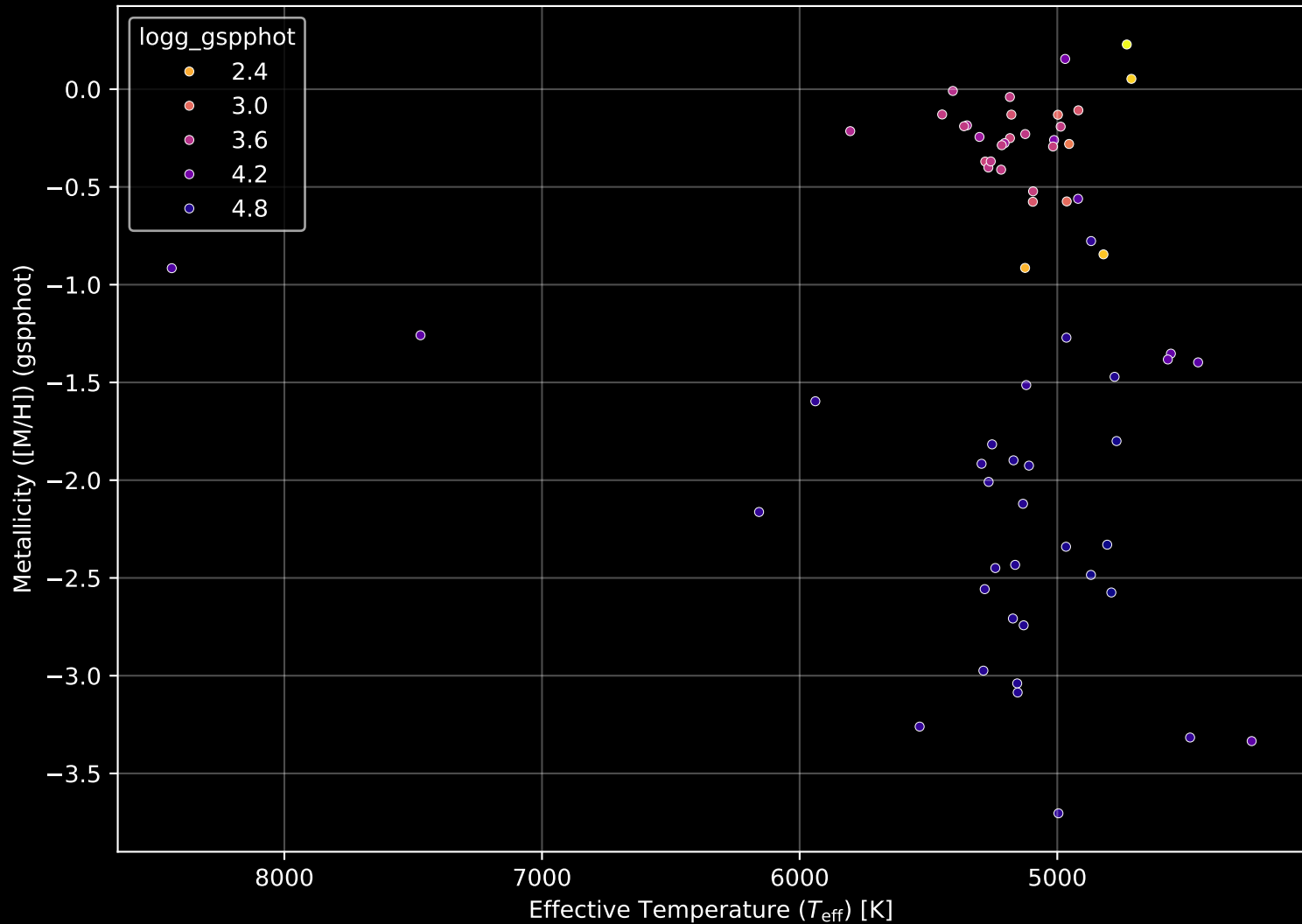
Gaia Cluster: [Berkeley_25] Stellar Population Parameters (n= 65)
