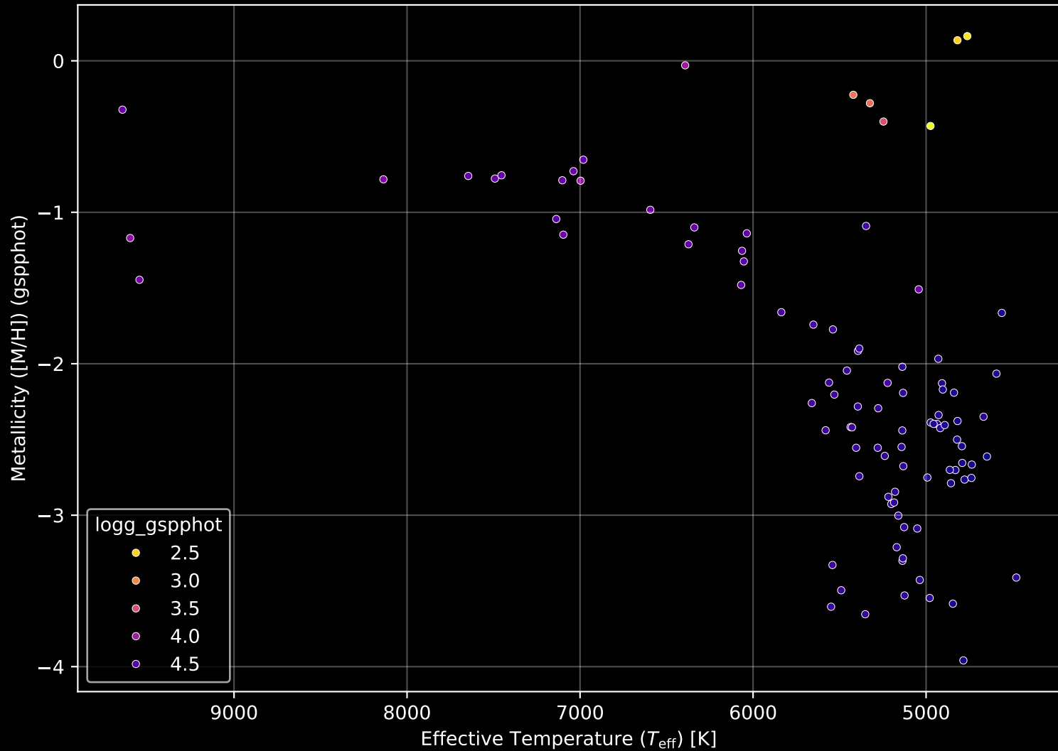
Gaia Cluster: [Berkeley_27] Stellar Population Parameters (n= 98)
