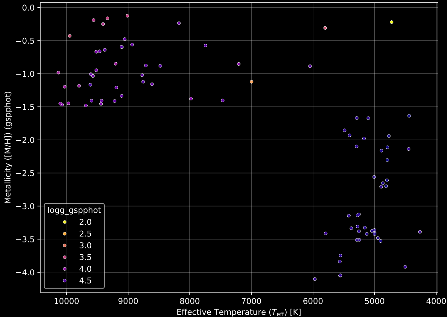
Gaia Cluster: [Berkeley_28] Stellar Population Parameters (n= 85)
