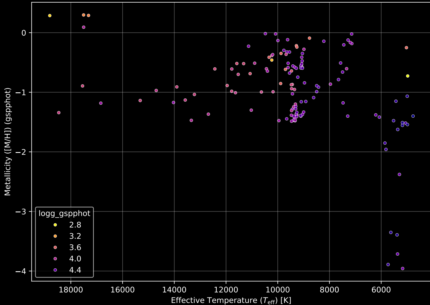
Gaia Cluster: [Berkeley_4] Stellar Population Parameters (n= 139)
