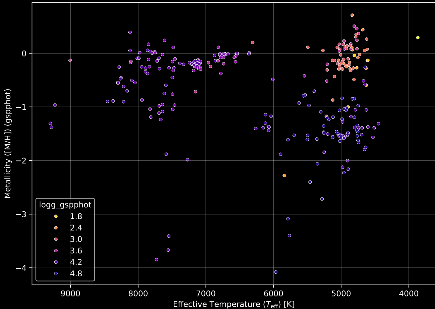
Gaia Cluster: [Berkeley_44] Stellar Population Parameters (n= 300)
