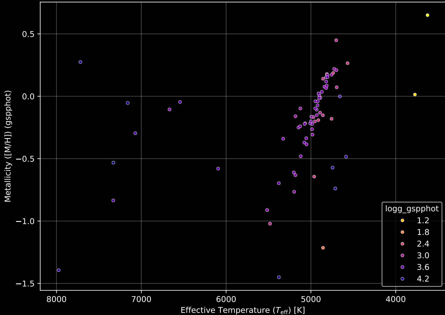
Gaia Cluster: [Berkeley_52] Stellar Population Parameters (n= 74)
