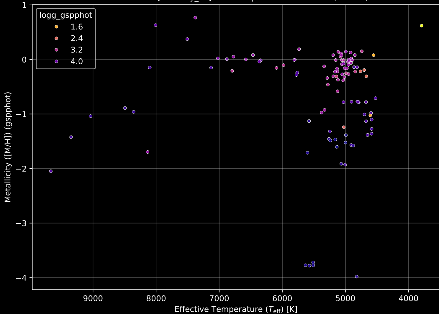
Gaia Cluster: [Berkeley_54] Stellar Population Parameters (n= 114)
