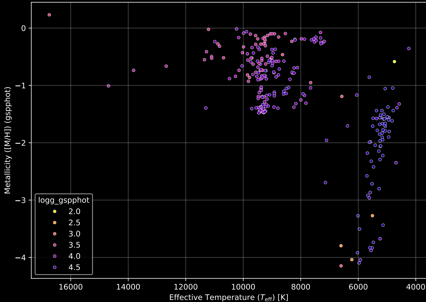
Gaia Cluster: [Berkeley_58] Stellar Population Parameters (n= 258)
