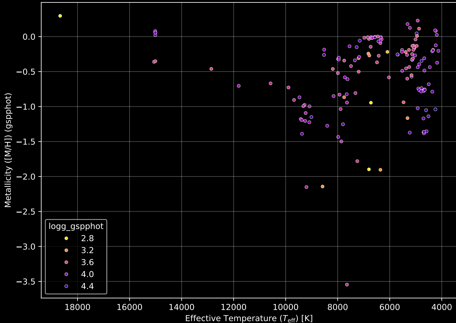
Gaia Cluster: [Berkeley_59] Stellar Population Parameters (n= 149)
