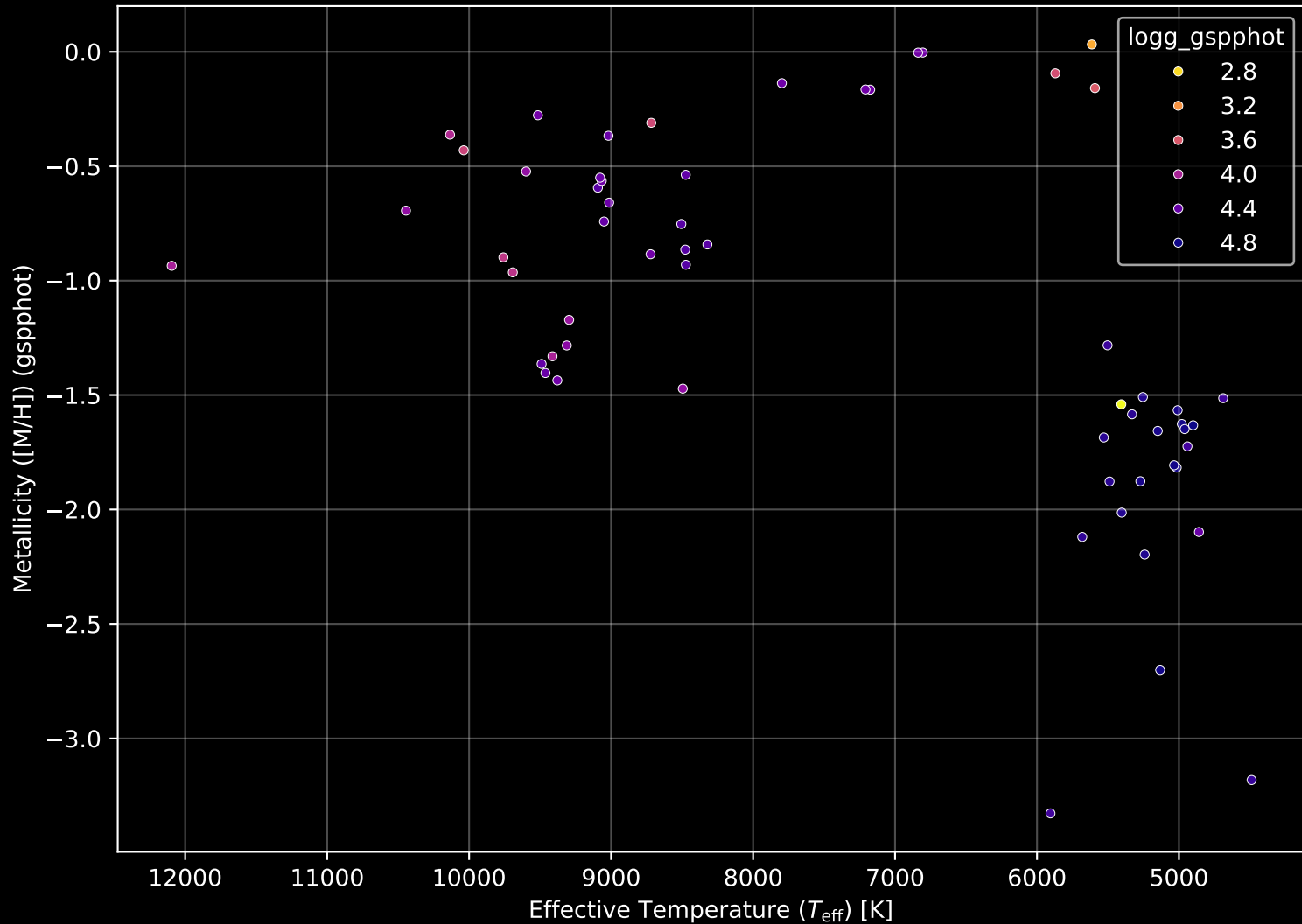
Gaia Cluster: [Berkeley_61] Stellar Population Parameters (n= 59)
