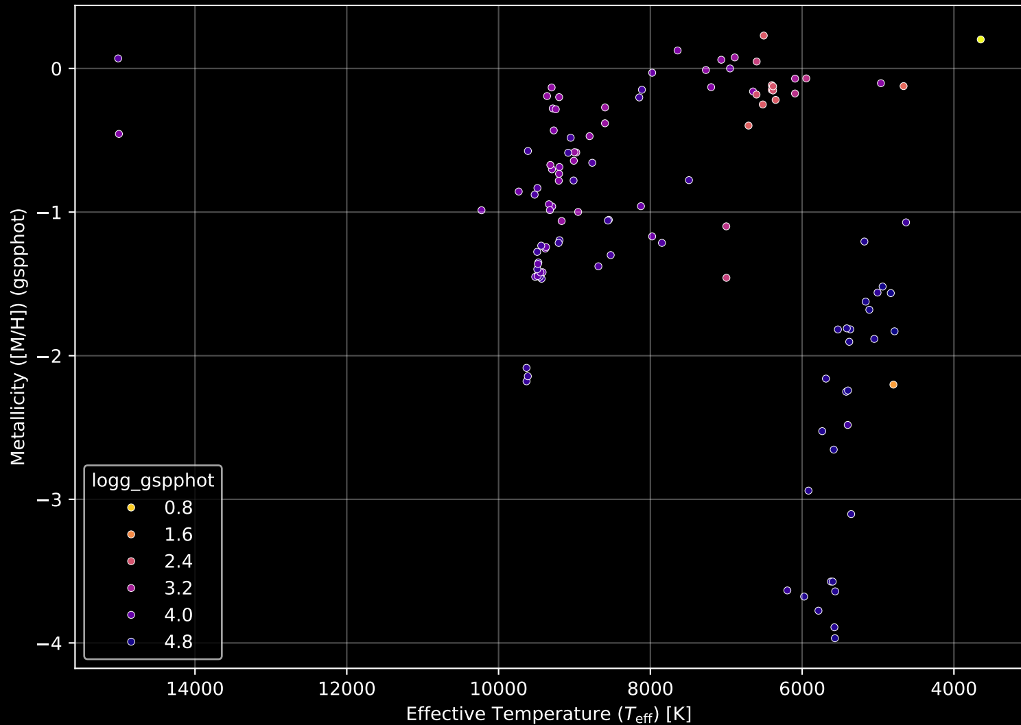
Gaia Cluster: [Berkeley_71] Stellar Population Parameters (n= 121)
