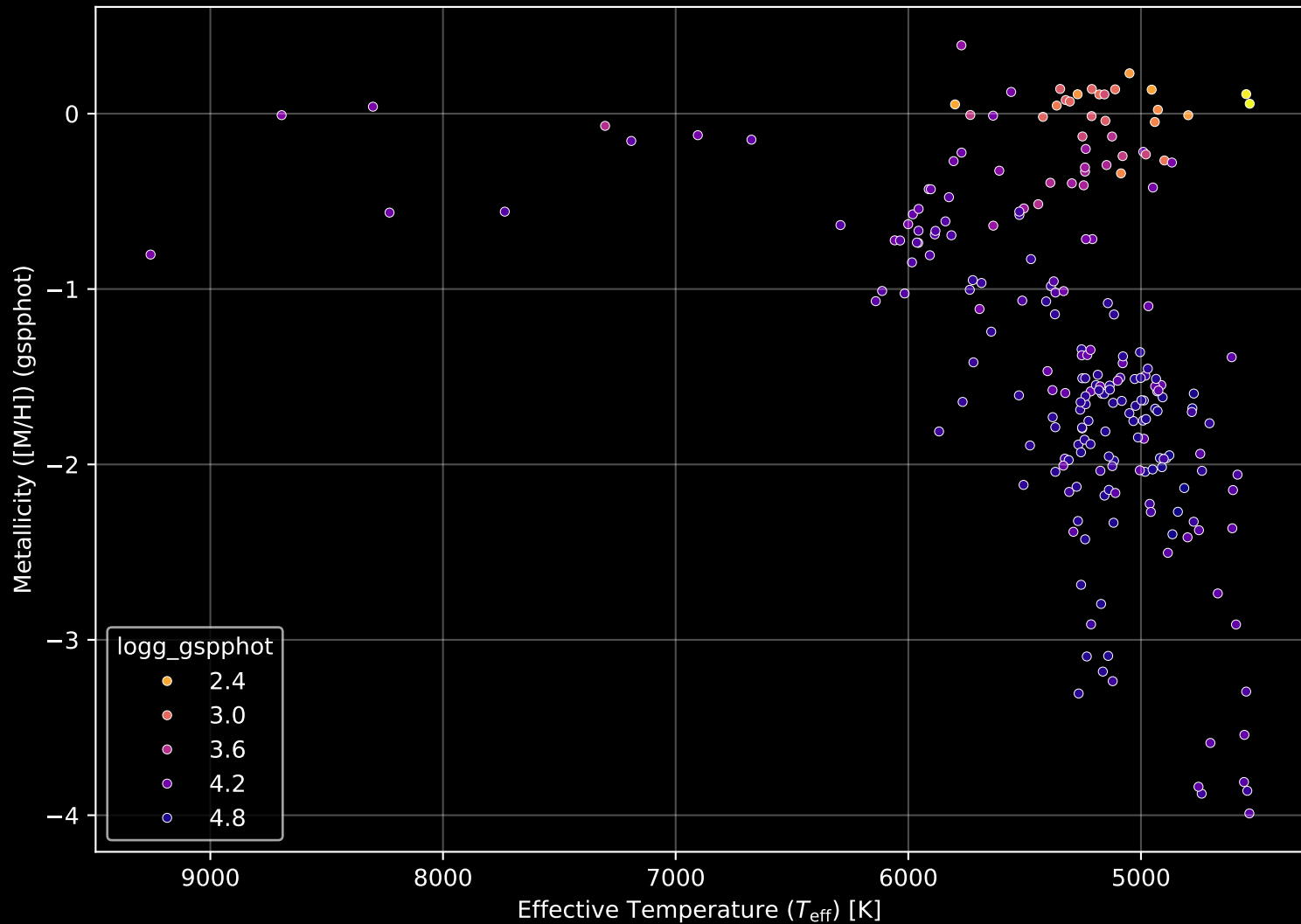
Gaia Cluster: [Berkeley_8] Stellar Population Parameters (n= 225)
