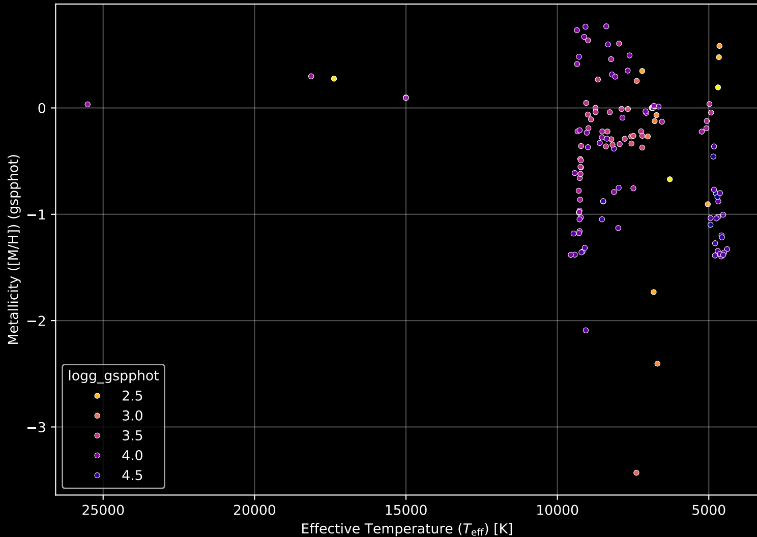
Gaia Cluster: [Berkeley_87] Stellar Population Parameters (n= 133)
