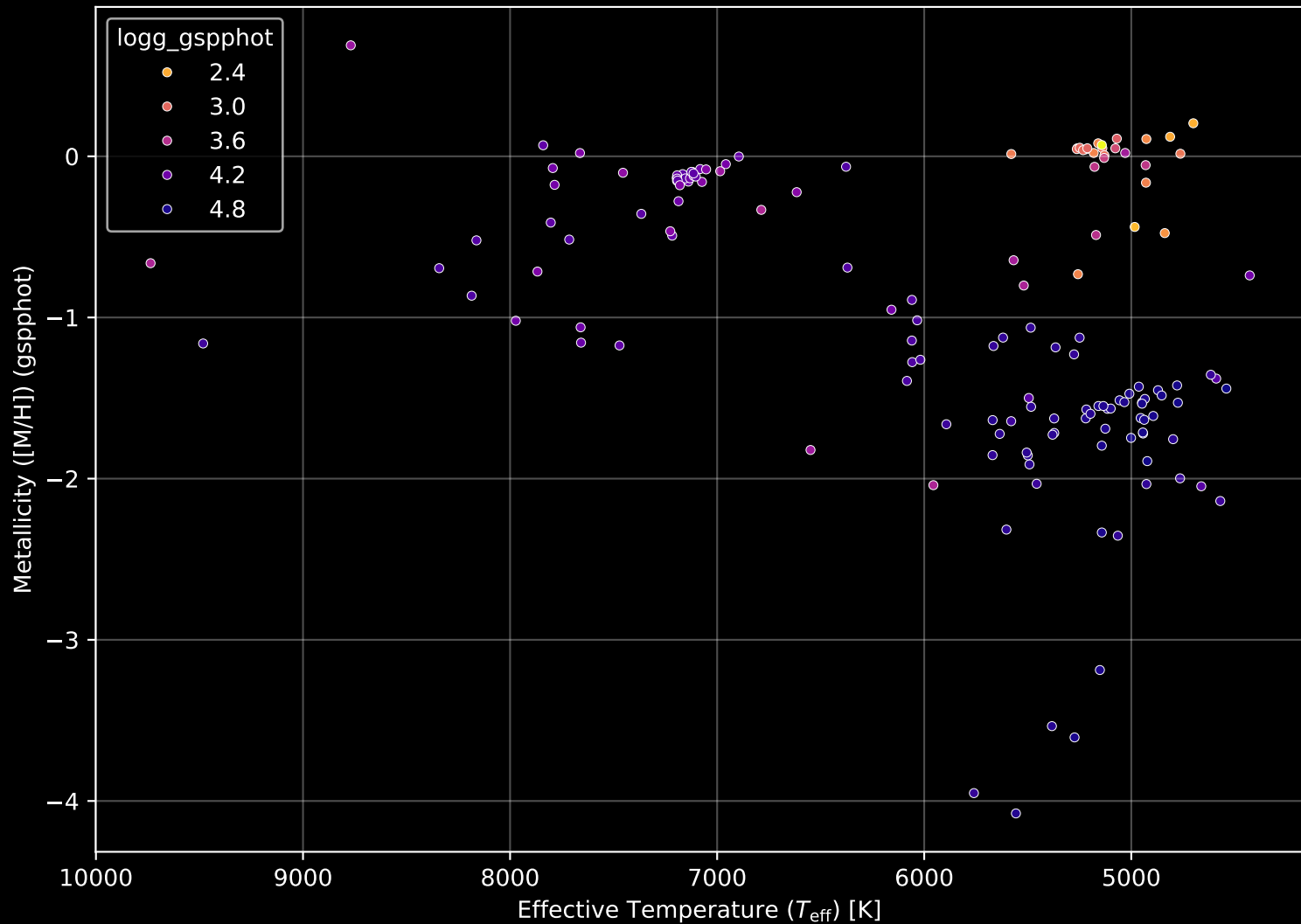
Gaia Cluster: [Berkeley_89] Stellar Population Parameters (n= 149)
