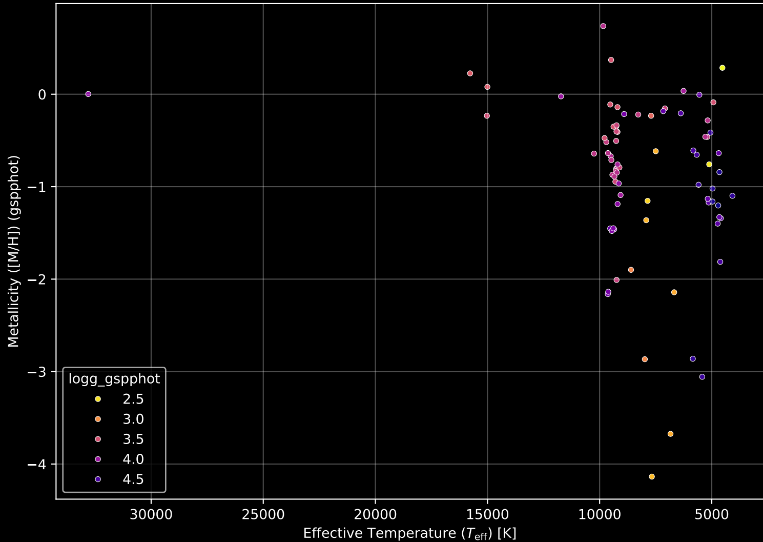
Gaia Cluster: [Berkeley_90] Stellar Population Parameters (n= 81)
