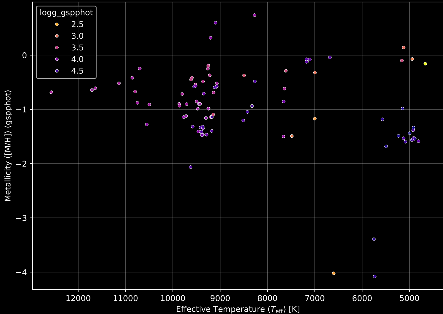
Gaia Cluster: [Berkeley_97] Stellar Population Parameters (n= 95)
