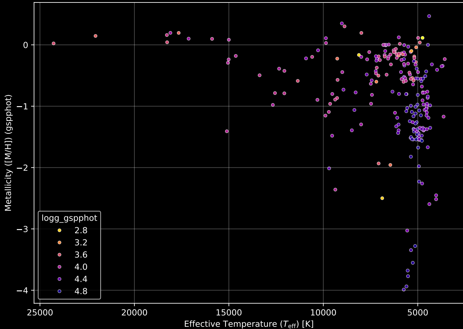
Gaia Cluster: [Biurakan_2] Stellar Population Parameters (n= 235)
