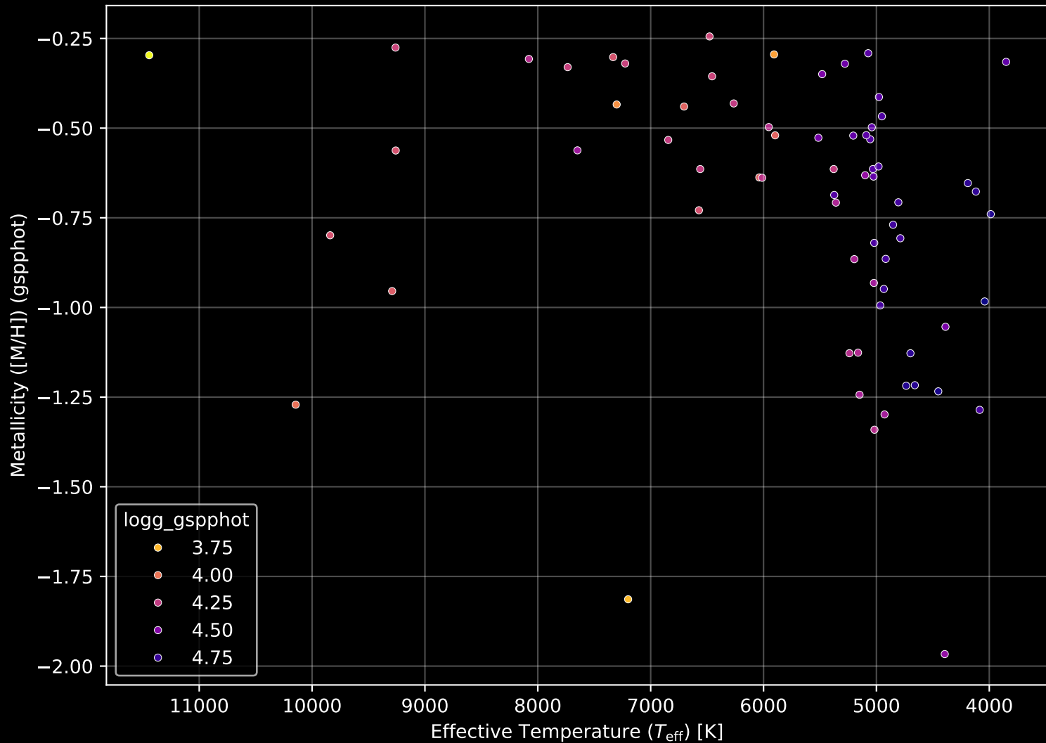
Gaia Cluster: [Bochum_4] Stellar Population Parameters (n= 68)
