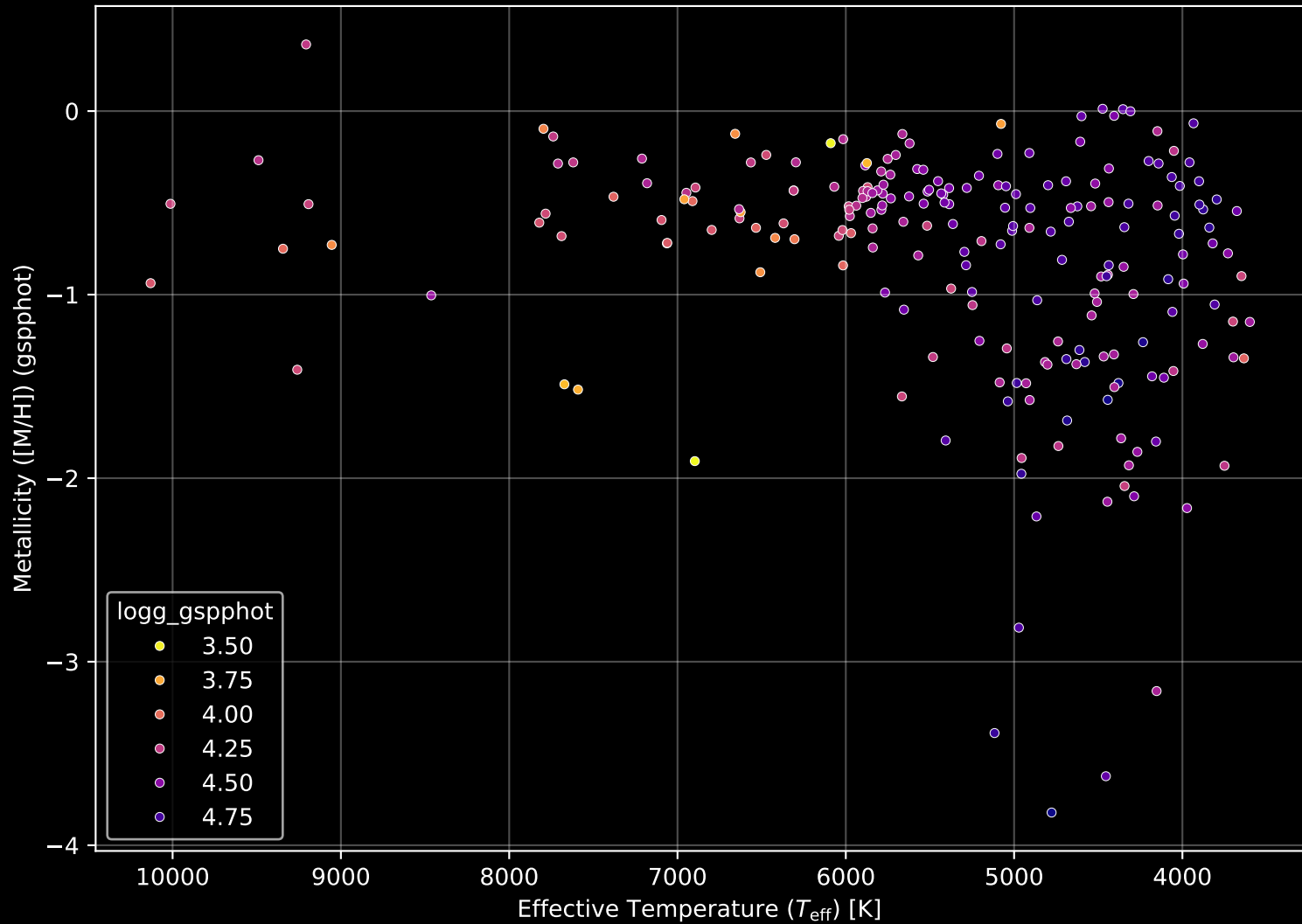
Gaia Cluster: [COIN-Gaia_24] Stellar Population Parameters (n= 220)
