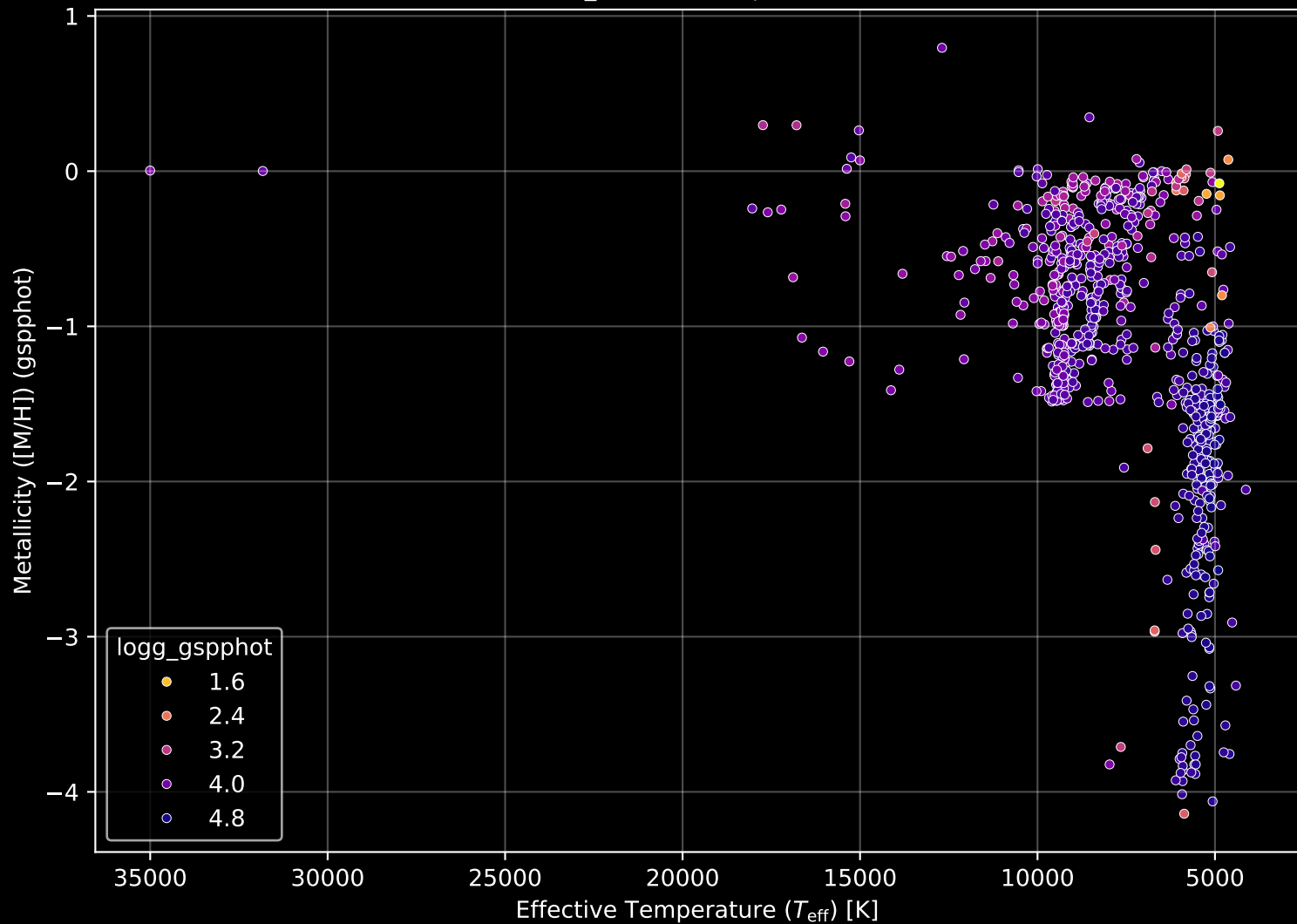
Gaia Cluster: [COIN-Gaia_29] Stellar Population Parameters (n= 830)
