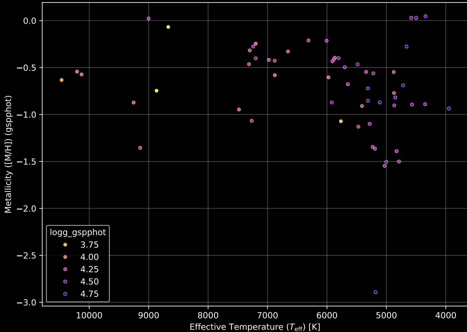
Gaia Cluster: [COIN-Gaia_34] Stellar Population Parameters (n= 58)
