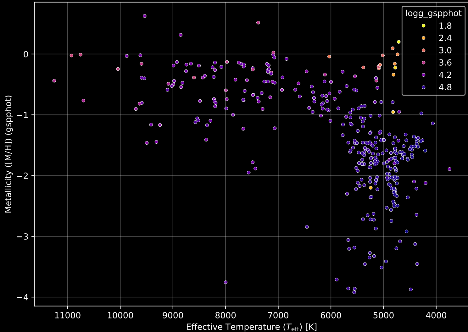
Gaia Cluster: [COIN-Gaia_40] Stellar Population Parameters (n= 360)
