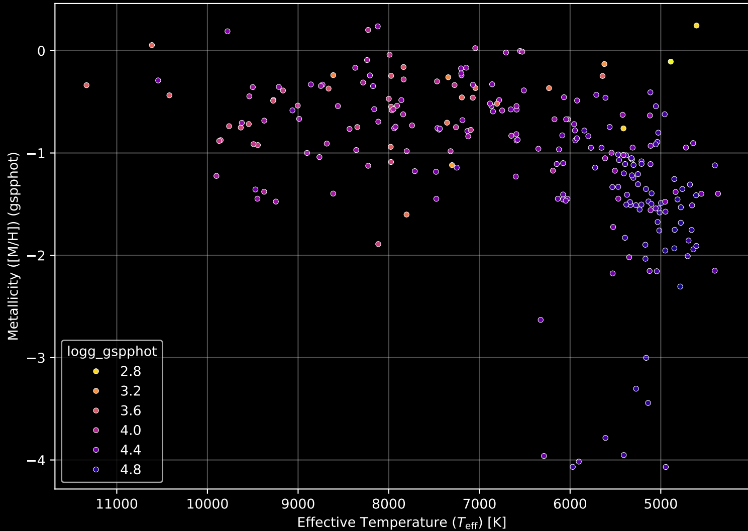
Gaia Cluster: [Collinder_220] Stellar Population Parameters (n= 245)
