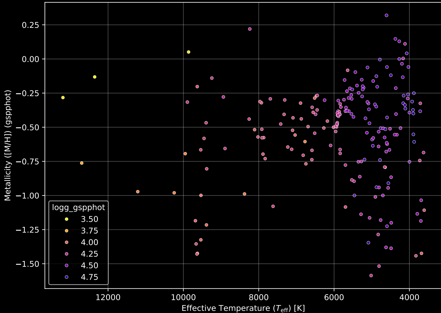
Gaia Cluster: [Collinder_394] Stellar Population Parameters (n= 208)
