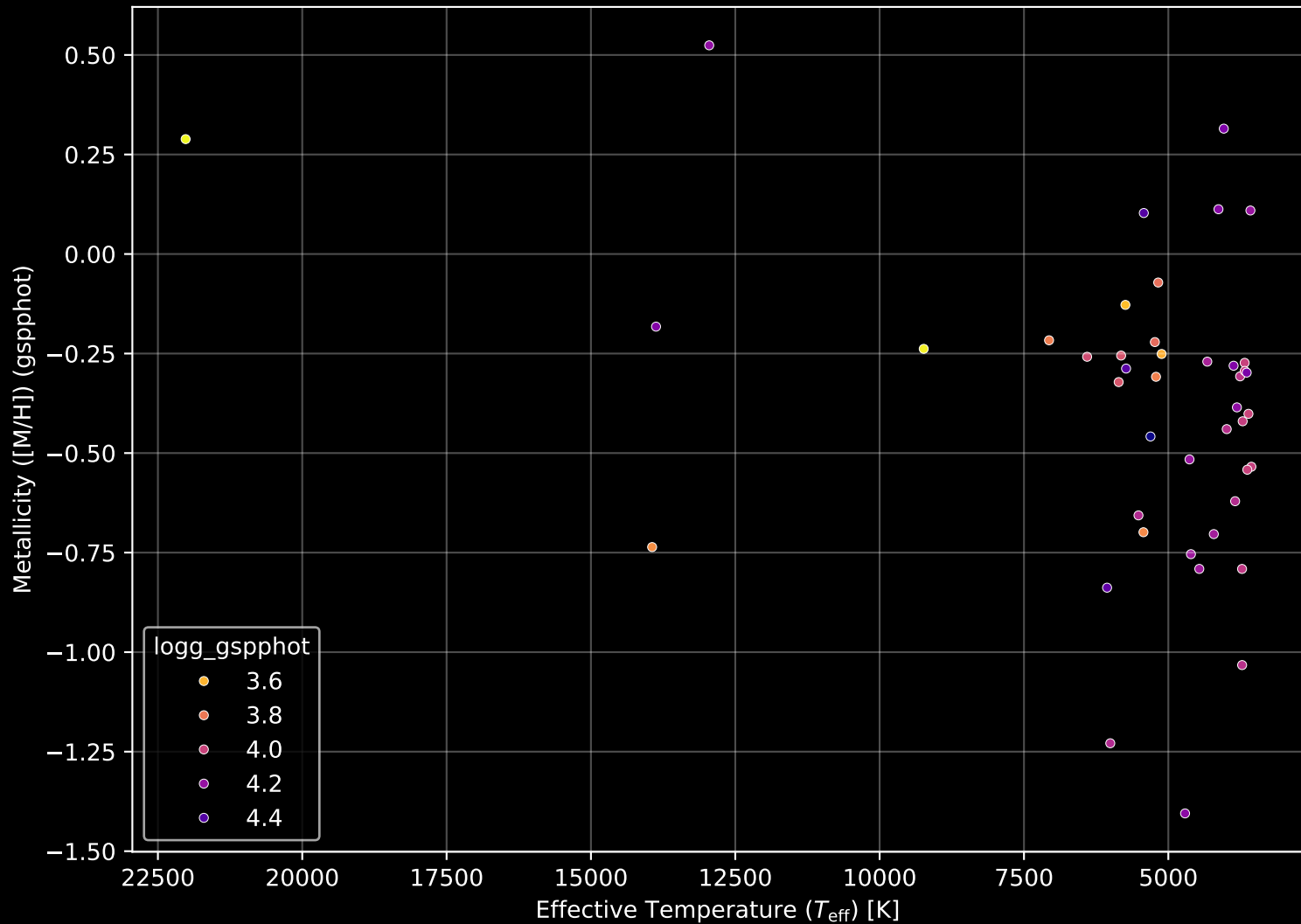
Gaia Cluster: [Collinder_419] Stellar Population Parameters (n= 44)
