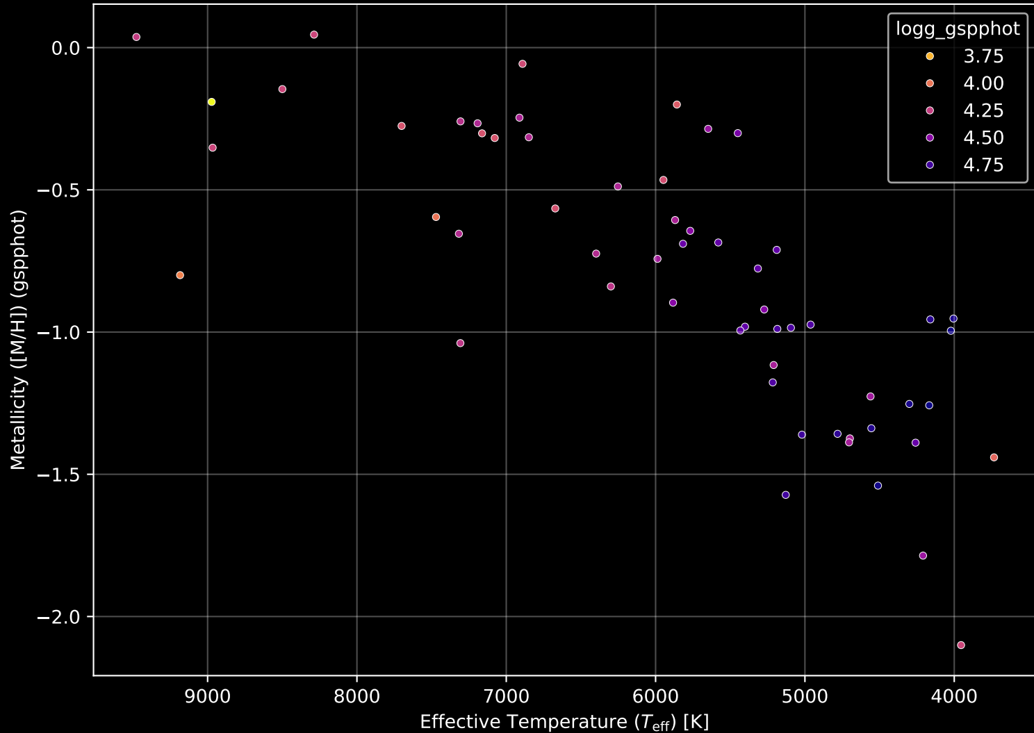
Gaia Cluster: [Czernik_18] Stellar Population Parameters (n= 58)
