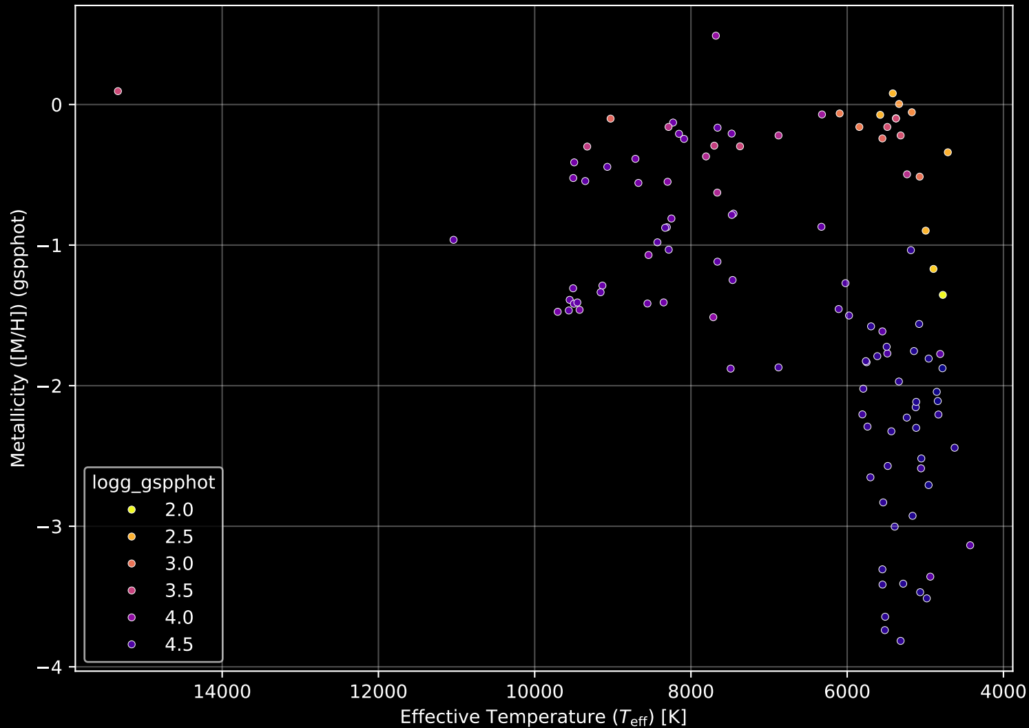
Gaia Cluster: [Czernik_20] Stellar Population Parameters (n= 113)
