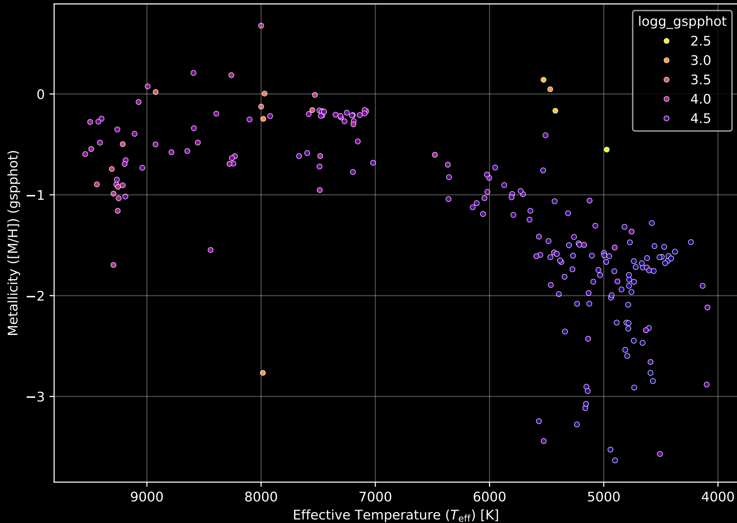
Gaia Cluster: [Czernik_25] Stellar Population Parameters (n= 199)
